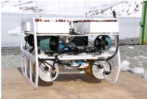
(a) ROV LUMA COPPE/UFRJ([6]).
