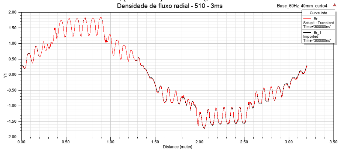
Figura 4-73 - densidade de fluxo radial, para a máquina em carga com curto na bobina #4
