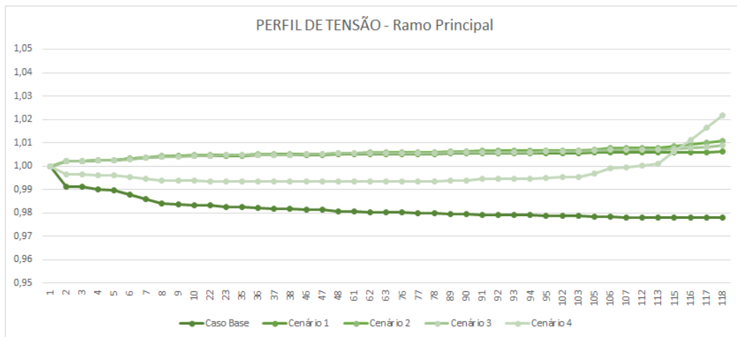
Figura 4.33: Sistema 134 barras - Perfil de tensão nas barras nos diferentes cenários - Ramo Principal
