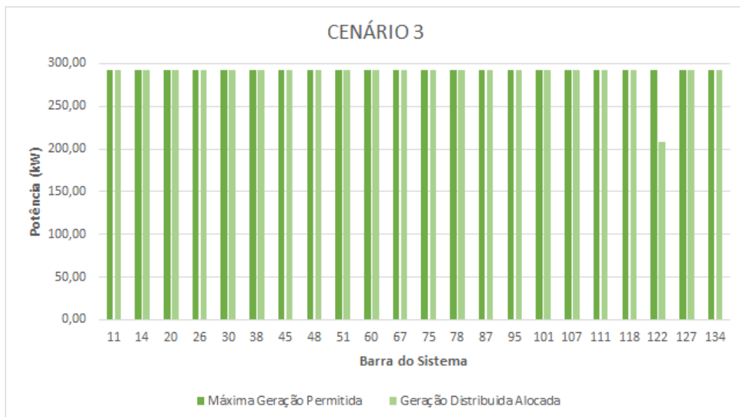
Figura 4.27: Sistema 134 barras - Conexão de GD na barra do meio e final dos ramos
