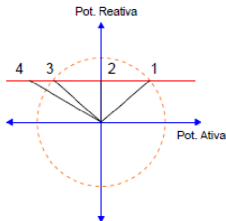
Figura 2.4: Modificação da Potência Aparente do Alimentador com a GD de fator de potência unitário
