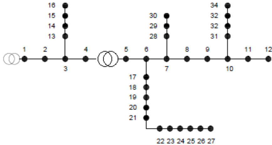
Figura 4.16: Diagrama unifilar do sistema de distribuição de testes do sistema 34 barras com regulador de tensão
